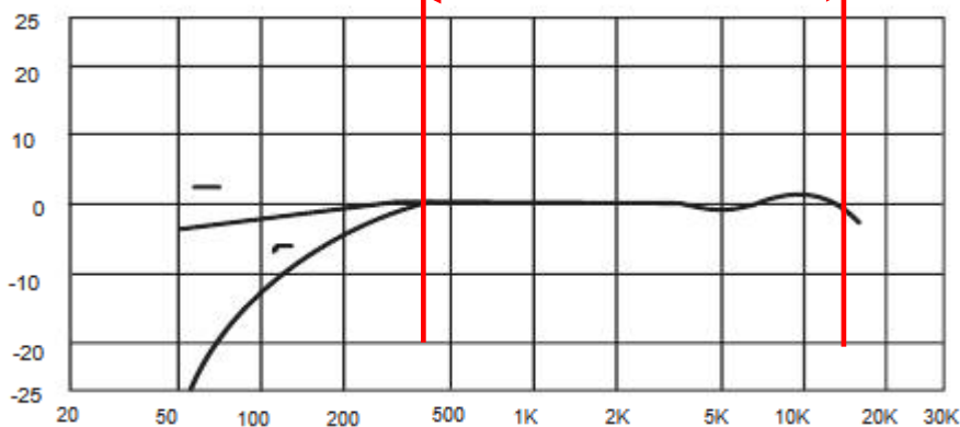
Frequenzdiagramm
