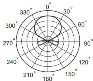
Polardiagramm @ 1kHz
